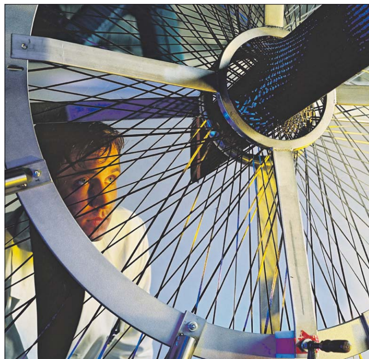
Automatisierte Produktion von Karbonfaserrohlingen durch einen Flechtroboter: Dabei werden bis zu 216 Kohlenstofffaserbündel rings um einen Kern angeordnet, so dass eine netzförmige Faserstruktur entsteht. Foto: Pressestelle EADS
