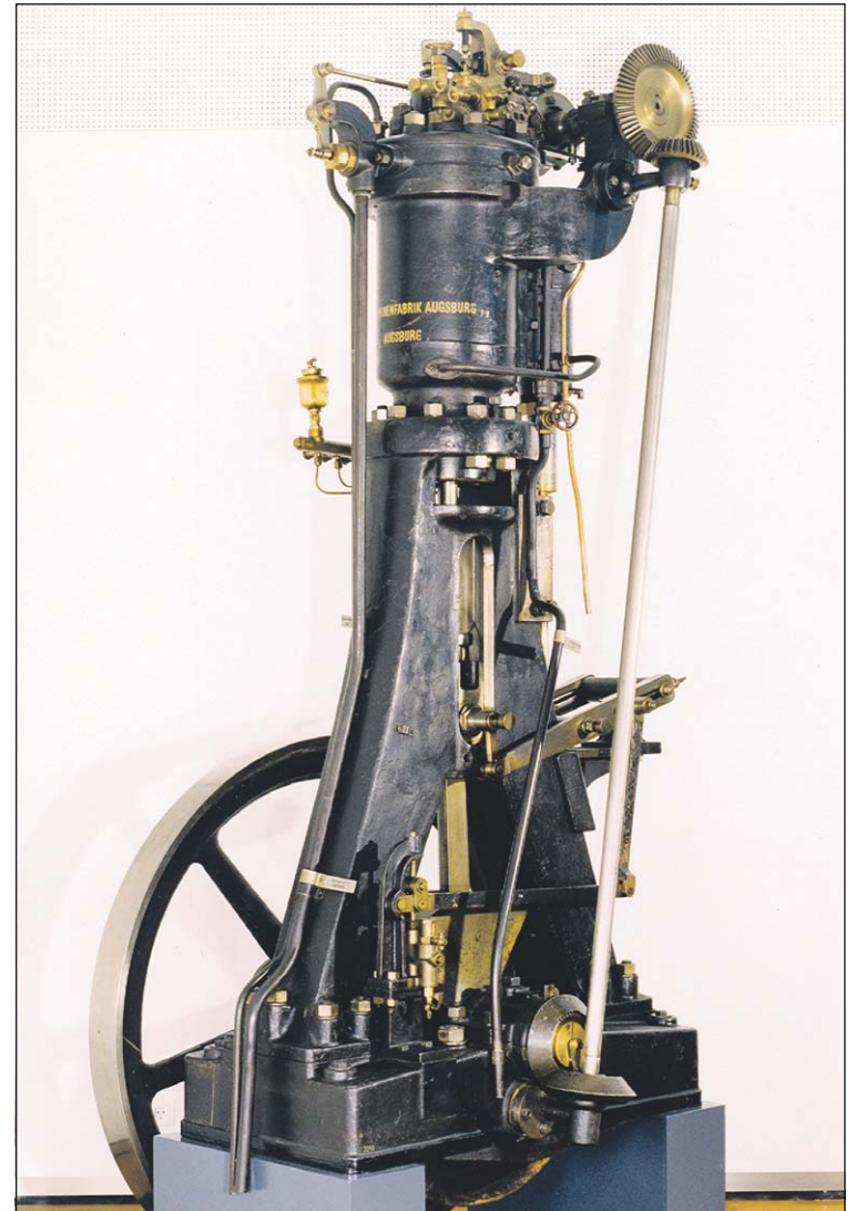
Rudolf Diesels Versuchsmotor aus der Maschinenfabrik Augsburg aus dem Jahr 1893.
